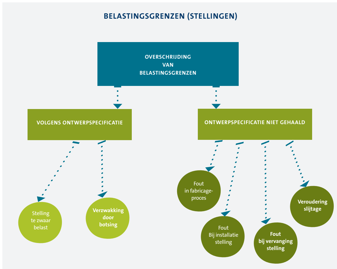
FIGUUR 2: VOORBEELD FOUTENBOOM VOOR Overschrijding BELASTINGSGRENZEN
